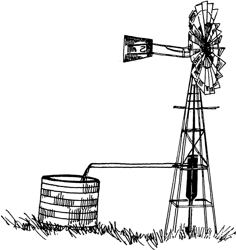
चित्र 24. दक्षिण अफ्रीका में पहाड़ी पर स्थापित एक पवन चालित पम्प जो अधिकतम वायुगति पर वायु ग्रहण करता है। भंडारण टैंक वायुरहित अवधि के लिए आवश्यक है।
