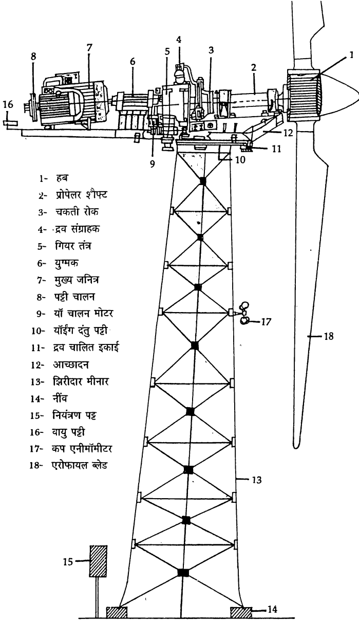
चित्र 16. एक आम पवन टर्बाइन।
