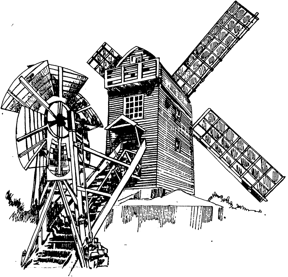
चित्र 9. सफाई की स्तंभ चक्की। पंखेनुमा पुच्छ स्तंभ खड़े दंड को चलाता है जो गियर के साथ छोटे 'ट्रक पहियों' से जुड़ा है। ट्रक पहिए एक गोलाकार पथ पर चलते हैं। अगल बगल से आने वाली हवाएं पंखेनुमा पुच्छ व पहियों को घुमाकर चक्की को वायु की दिशा में स्थापित कर देती हैं।
