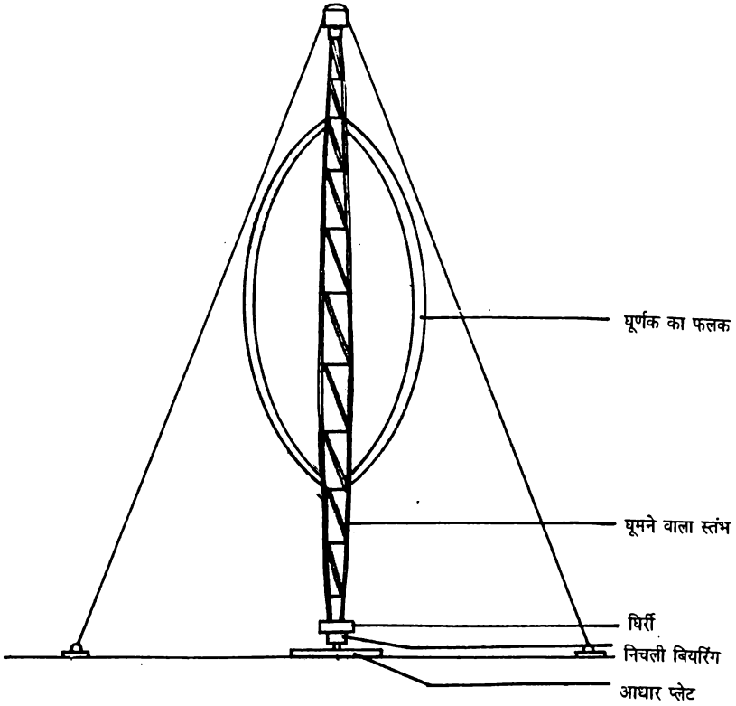
चित्र 23. एक ऊर्ध्व-अक्षीय घूर्णक तथा उसके विभिन्न घटक ।
