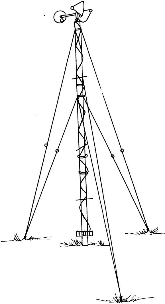
चित्र 26. कप वायुगति-मापक ।
