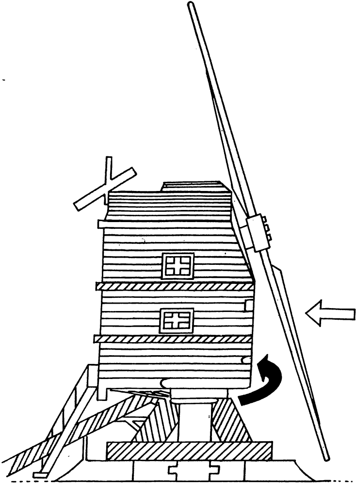
चित्र 2. यूरोप में एक स्तंभ चक्की।
