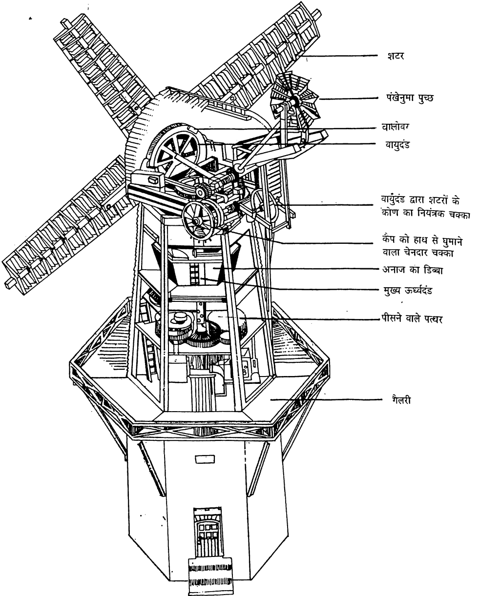
चित्र 13. एक पवन चक्की की संरचना। इसके कुछ खास-खास भाग भी दिखाए गए हैं।
