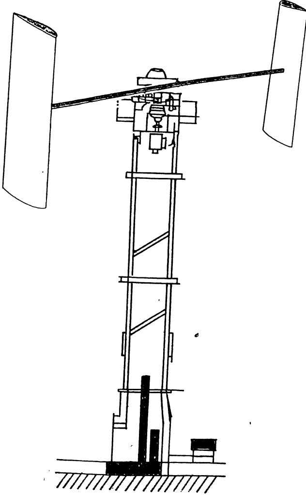
चित्र 20. एक उच्च गतिक, संशोधित ऊर्ध्व-अक्षीय पवन चक्की।
